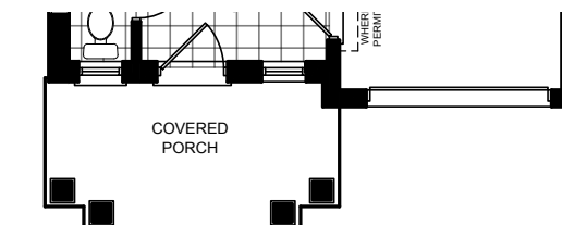
ELEV. B
