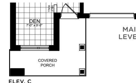
ELEV. C
