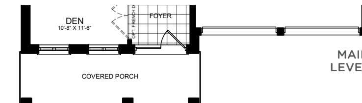
ELEV. B
