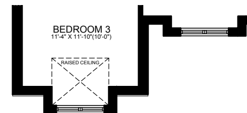
ELEV. B
