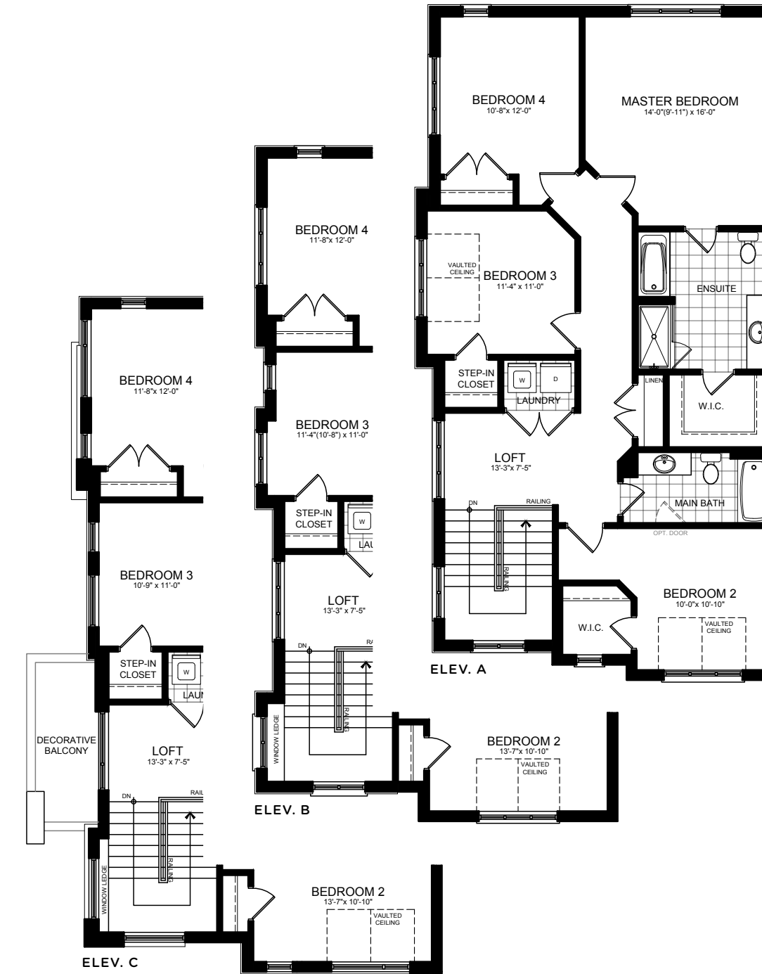
OPTIONAL 4 BEDROOM PLAN
